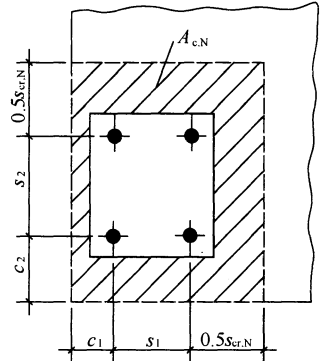
图 6.1.5-4 四栓受拉，位于构件角部的计算面积示意
