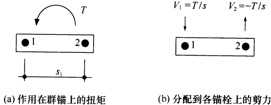
图 6.1.27-1 锚栓所受剪力方向相反示意
