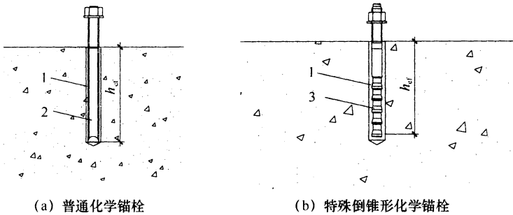
图 A.1.4 化学锚栓示意
