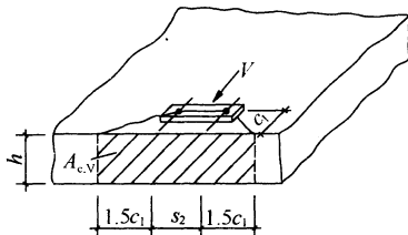
图 6.1.18-2 双栓受剪， 位于构件边缘示意
