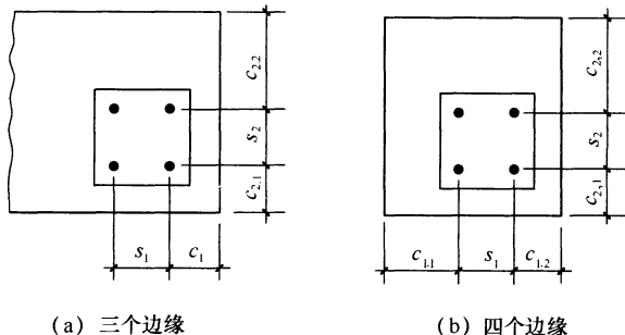
图 6.2.12 有多个边缘影响的群锚示意
