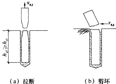
图 A.2.1 锚固钢材破坏示意
