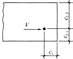
图 6.2.21 有多个边缘影响的锚栓示意
