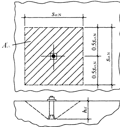
图 6.1.4 理想锥体破坏投影面面积示意
