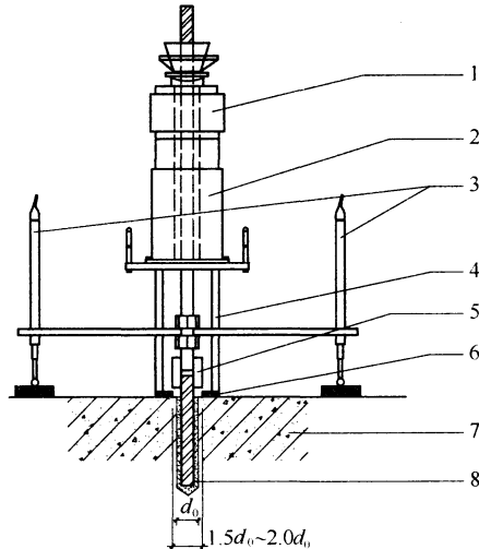
图 B.1.2 约束抗拉试验装置示意
